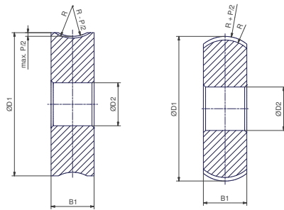
konkave / konvexe Rändelränder – Nr. 80
